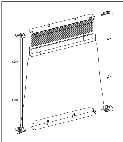
Mosquitera con guías laterales e inferior
