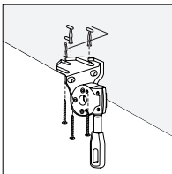
Taladrar y atornillar Soporte B
