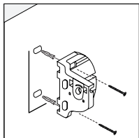
Taladrar y atornillar Soporte A
