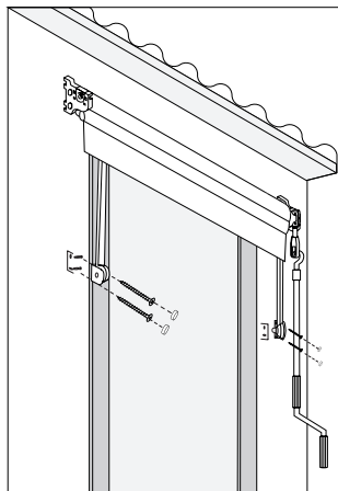
Taladrar y atornillar
