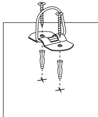
Fijar
