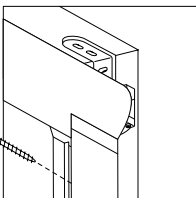
Fijar
