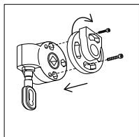
Girar y atornillar
